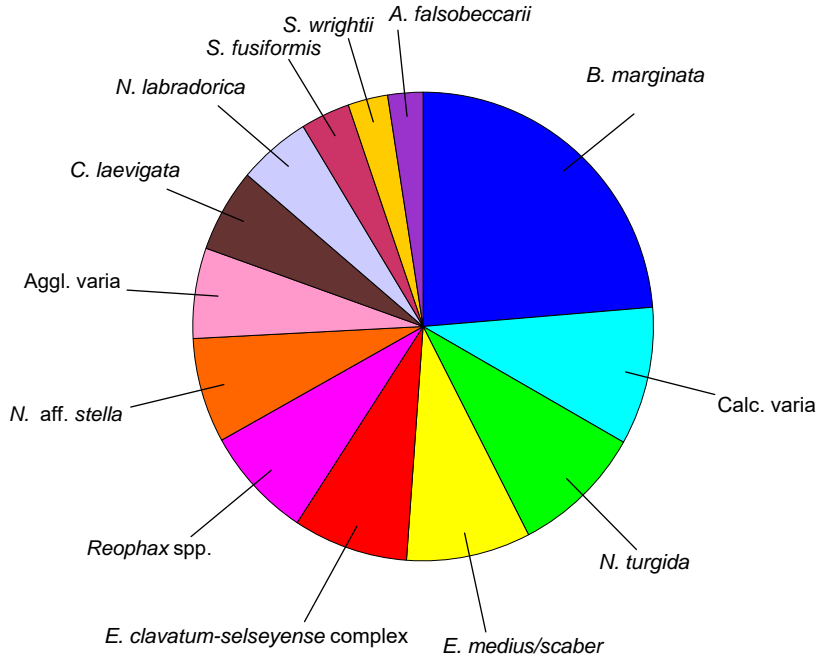
Anholt, Kattegat (Total (live+dead) C-An-1a)
