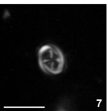
S. cf. laffittei W-7, 730
