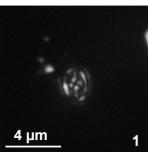
S. handleyi W-3, 30
