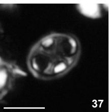
C. trabalis W-4, 168
