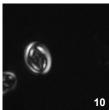
S. ourmae sp. nov. W-6, 969
