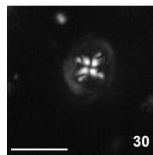
C. bifarius W-3, 30
