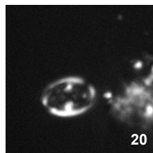
S. cf. ngurumahambaensis W-3, 594
