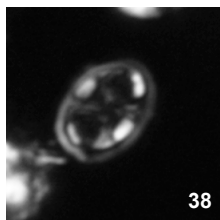
C. trabalis W-4, 168
