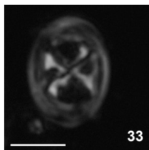
C. litterarius W-4, 274
