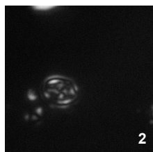
S. handleyi W-3, 30
