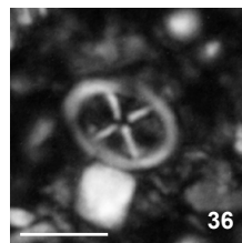
C. synquadriferforatus W-8, 681
