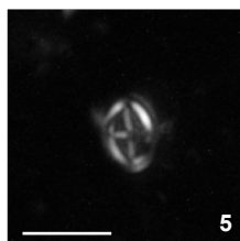
S. cf. handleyi W-7, 910
