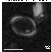
L. armilla W-5, 755
