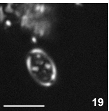
S. cf. ngurumahambaensis W-3, 594
