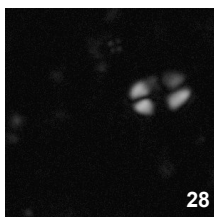
O. terrazetus W-4, 307.84
