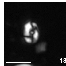
M. keadyi W-5, 755
