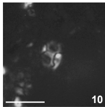
O. hillii W-4, 1120.14
