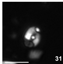
R. laswellii W-5, 755
