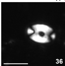
R. bukryi W-5, 755
