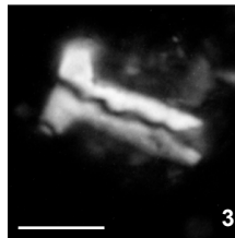
L. maleformis W-7, 1000m
