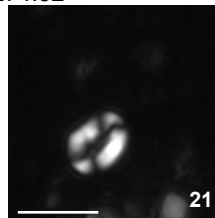
M. lesliae W-5, 755
