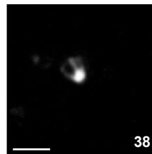
D. leariae W-7, 730
