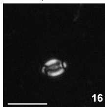
cf. Bil. wadeae W-6, 969
