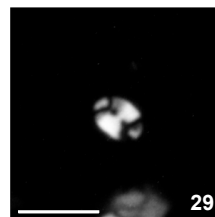
O. cf. terrazetus W-7, 730
