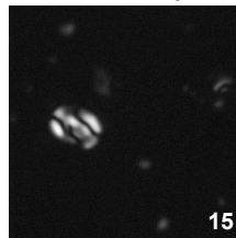
Bil. wadeae W-4 274.32
