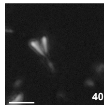
N. baileyi W-4, 835.15
