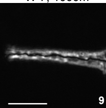
L. cayeuxii W-4 274.32
