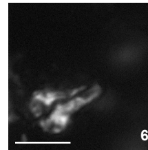
L. cf. maleformis W-2, 2293.6
