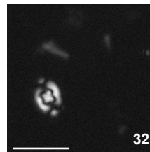
cf. R. laswellii W-4, 646.18
