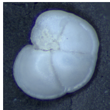
Globorotalia menardii
