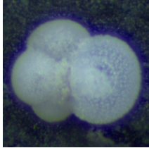
Globigerinita glutinata
