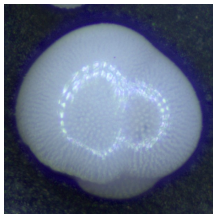
Pulleniatina obliquiloculata
