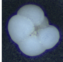
Neogloboquadrina dutertrei
