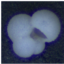
Globigerina bulloides
