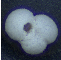
Globigerinoides ruber
