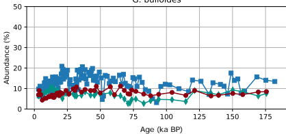
G. bulloides
