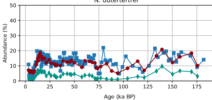
N. dutertrei
