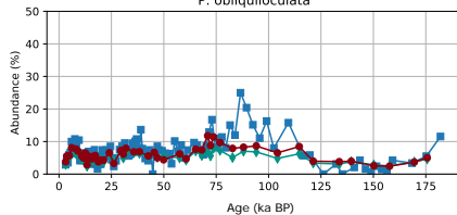
P. obliquiculata
