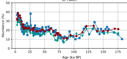
G. ruber
