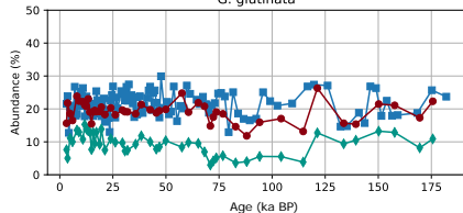
G. glutinata
