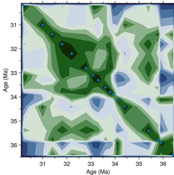
d ODP 689D
