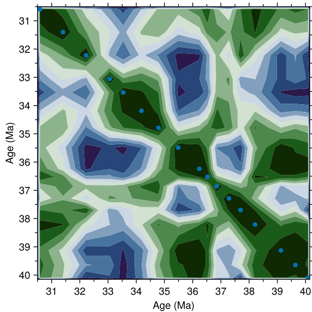
c ODP 748B
